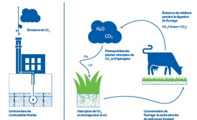
LE CYCLE DU CARBONE
