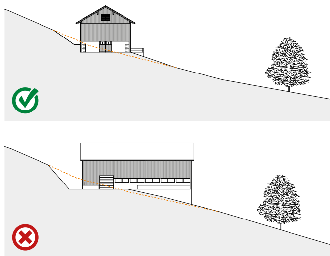
Illustration 4: Bâtiments construits avec et contre la topographie. Dans l'exemple réussi, en haut, la grange est orientée de façon longitudinale par rapport à la pente. Les grands volumes du bâtiment n'apparaissent pas d'une hauteur excessive côté aval. Dans le mauvais exemple, en bas, la grange est orientée dans le prolongement de la pente. La façade aval apparaît clairement trop haute. 5
